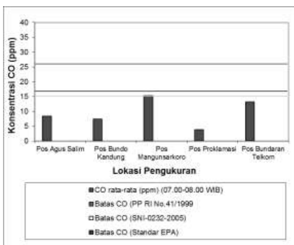
Gambar 21. Tingkat Konsentrasi Rata-rata CO di Pos Polisi Lalu Lintas
