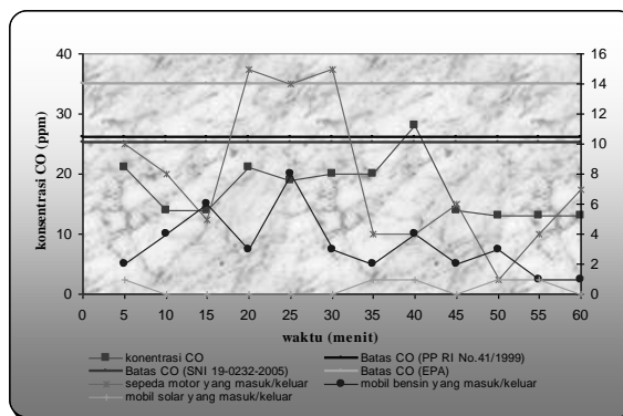
Gambar 6. Perubahan Konsentrasi CO pada Jam 14.35-15.35 WIB di Areal Parkir Rocky Plaza Hotel Tanggal 1 Oktober 2006 (Titik 3)
