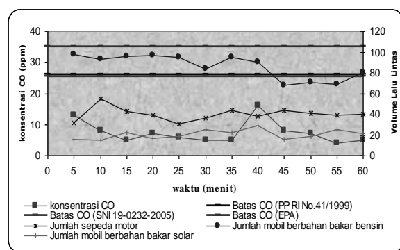
Gambar 17. Perubahan Konsentrasi CO Selama 1 Jam Pengukuran di Pos Bundo Kandung pada jam 14.00-15.00 WIB
