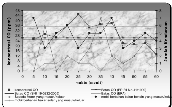
Gambar 10 Perubahan Konsentrasi CO pada Jam 11.30-12.30 WIB di Areal Parkir Plaza Andalas (Titik 4)
