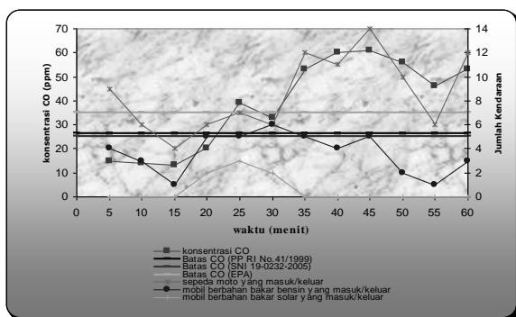
Gambar 4. Perubahan Konsentrasi CO pada Jam 11.30-12.30 WIB di Areal Parkir Rocky Plaza Hotel Tanggal 1 Oktober 2006 (Titik 1)
