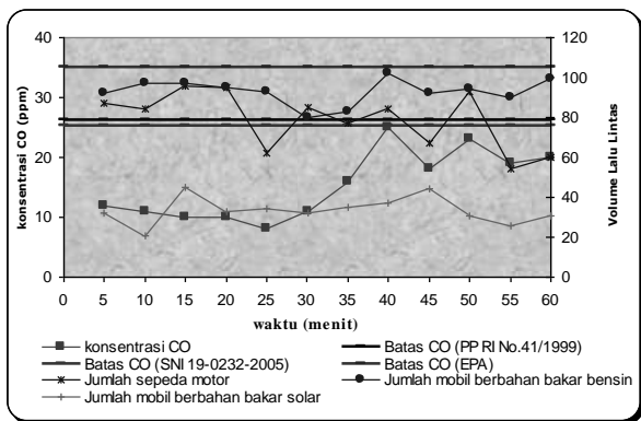
Gambar 18. Perubahan Konsentrasi CO Selama 1 Jam Pengukuran di Pos Mangunsarkoro pada jam 07.20-08.20 WIB
