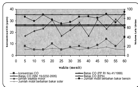
Selama 1 Jam Pengukuran di Pos Agus Salim.
