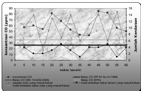
Gambar 5. Perubahan Konsentrasi CO pada Jam 13.30-14.30 WIB di Areal Parkir Rocky Plaza Hotel Tanggal 1 Oktober 2006 (Titik 2)
