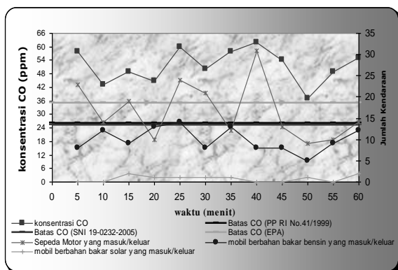
Gambar 9. Perubahan Konsentrasi CO pada Jam 16.30-17.30 WIB di Areal Parkir Plaza Andalas (Titik 3)
