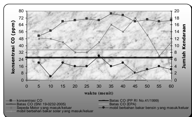
Gambar 8 Perubahan Konsentrasi CO pada Jam 15.00-16.00 WIB di Areal Parkir Plaza Andalas (Titik 2)
