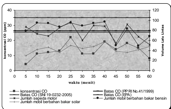
Gambar 20. Perubahan Konsentrasi CO Selama 1 Jam Pengukuran di Pos Simpang Telkom pada jam 07.30-08.30 WIB
