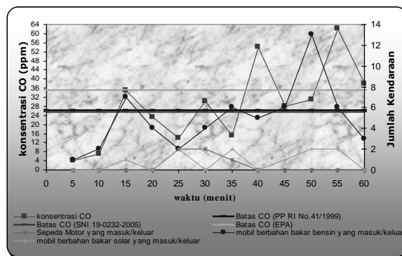
Gambar 11. Perubahan Konsentrasi CO pada Jam 13.00-14.00 WIB di Areal Parkir Plaza Andalas (Titik 5)
