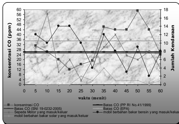
Gambar 7 Perubahan Konsentrasi CO pada Jam 14.00-15.00 WIB di Areal Parkir Plaza Andalas (Titik 1)
