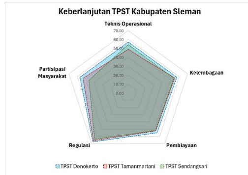
Gambar 11 Status Keberlanjutan Seluruh Aspek pada TPST di Kabupaten Sleman
